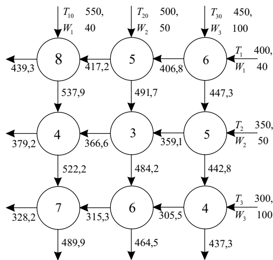
Рис. 2. Структура системы многопоточного теплообмена.
