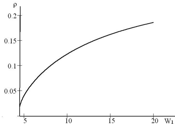
Рис. 1. Зависимость показателя термодинамического совершенства теплообменника смешения от водяного эквивалента W_1 .
